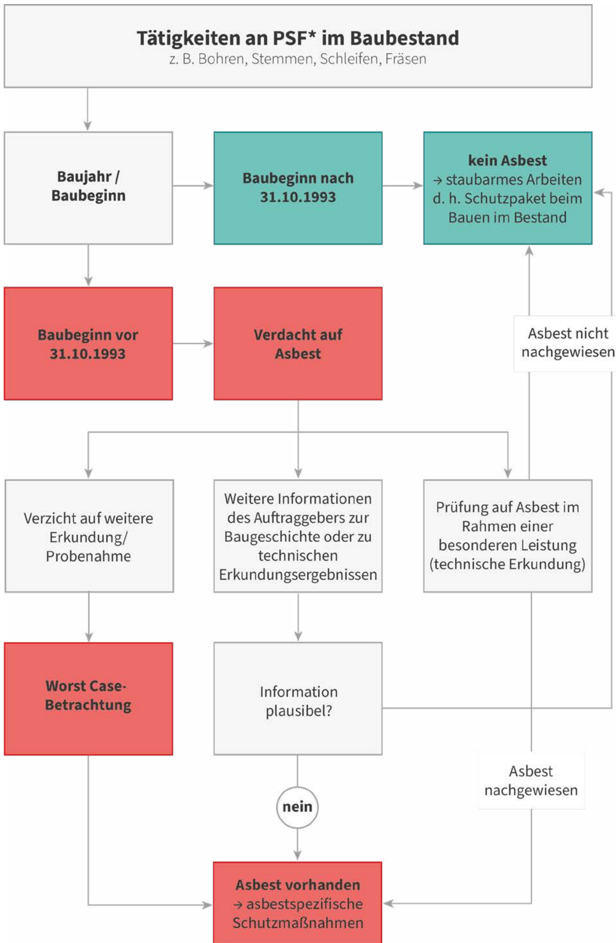
Abb. 7: Vorgehen bei Tätigkeiten mit potenziell asbesthaltigen PSF* beim Bauen im Bestand
